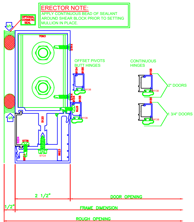
822 O.G. JAMB 5600 6"
