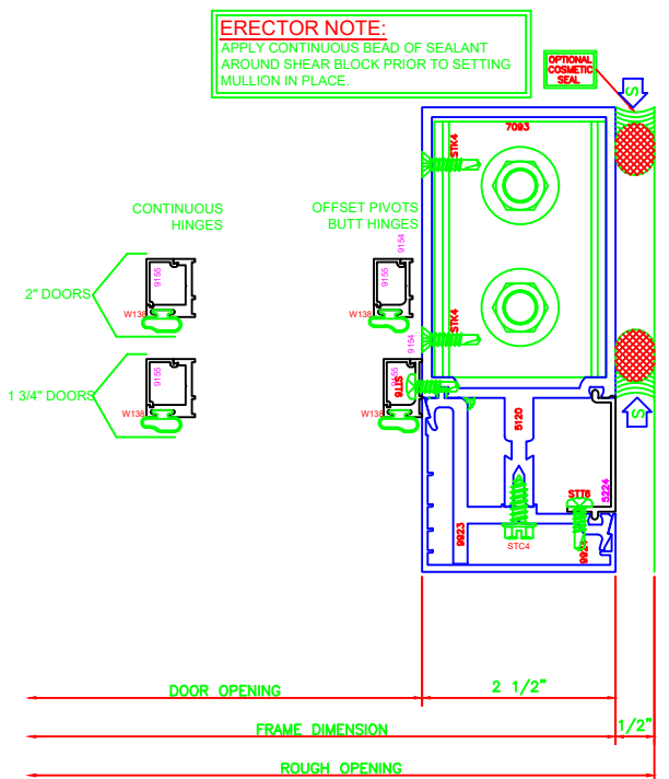
823 O.G. JAMB 5600 6"
