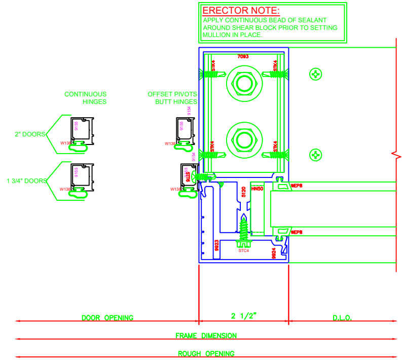
823 O.G. JAMB 5600 6"
